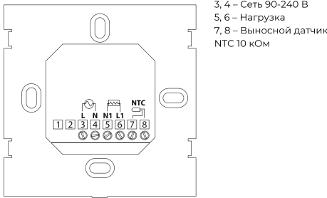
Схема подключения
