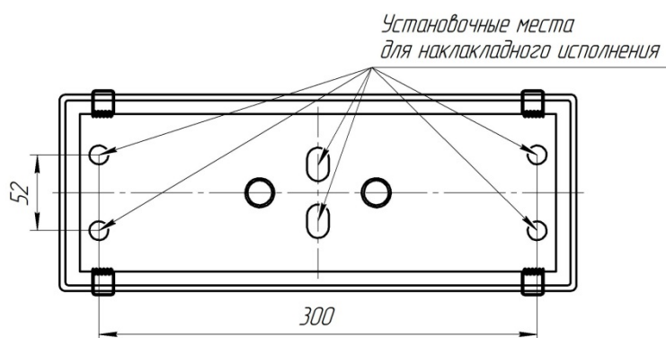
Рис. 1. Габаритные размеры
