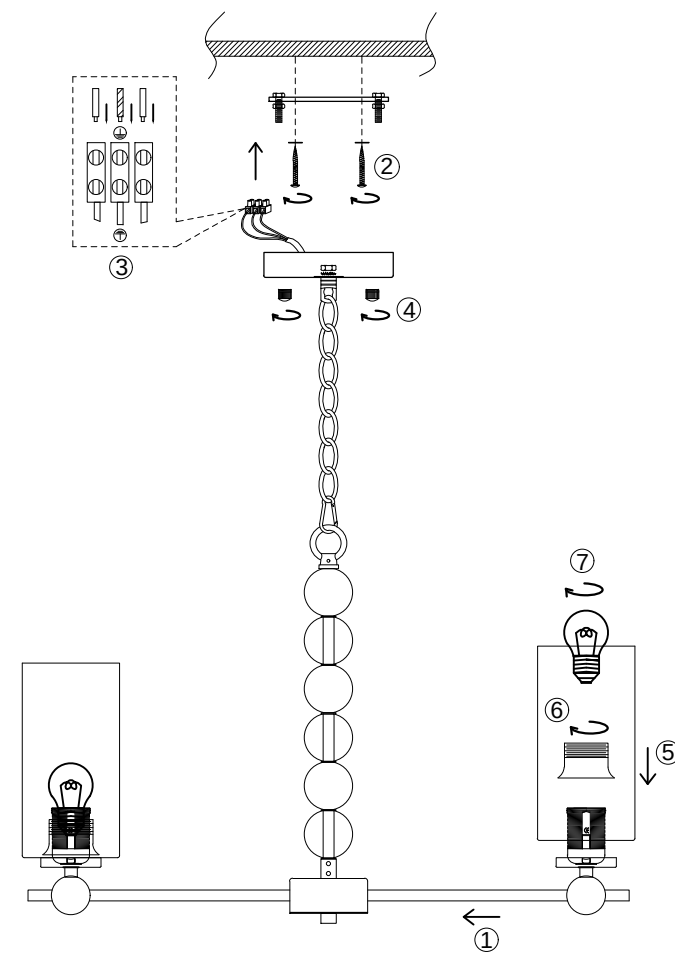
Подвесной светильник E27 40W
