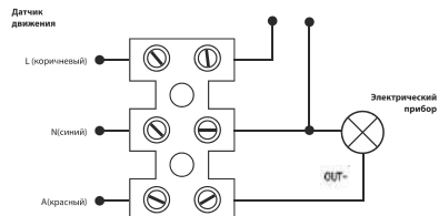
Рис. 2 Схема электропитания
