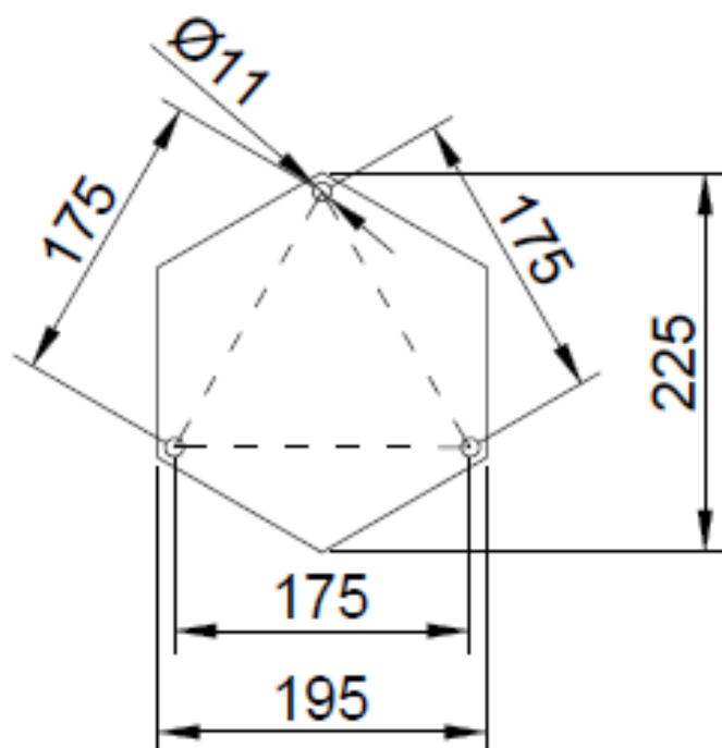
Схема основания светильника PL766
