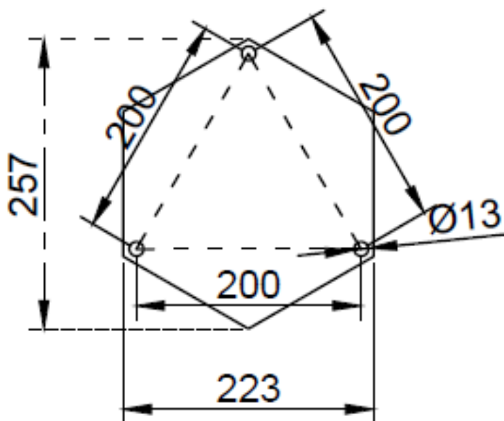
Схема основания светильника PL767
